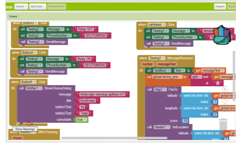
Figure 10. MIT App Inventor Block
